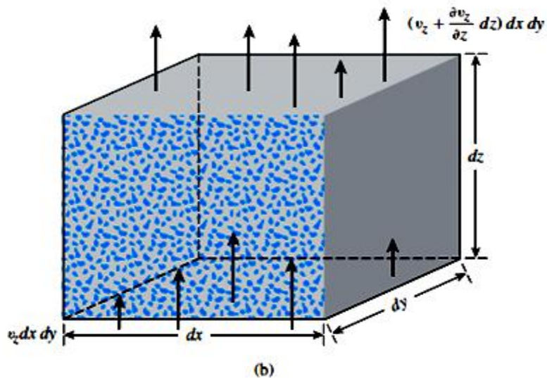
Figura 4.3 (a) Shtresa e argjilës që i nënshtrohet konsolidimit i (b) Rrjedhja e ujit në pikën A gjatë konsolidimit
