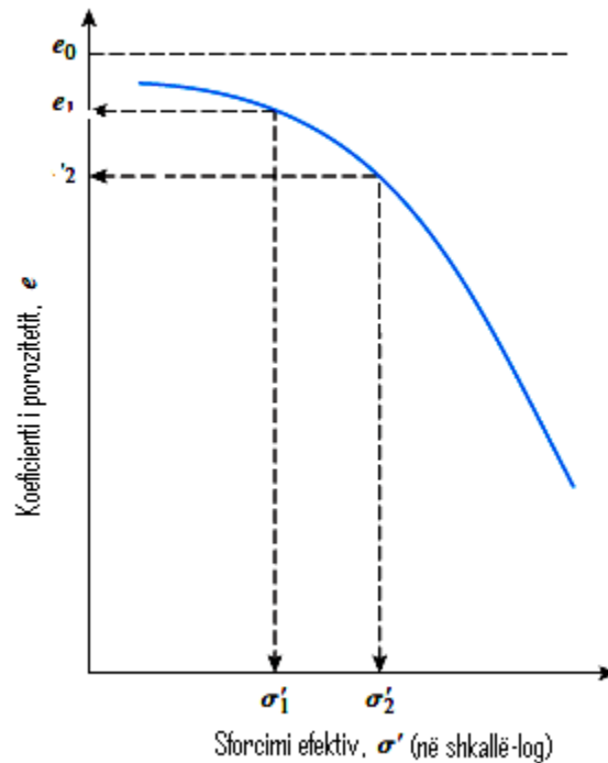
Figura 3.10 Diagrami tipik i bashkëlidhjes e - \log \sigma' ( e kundrejt \log \sigma' )
