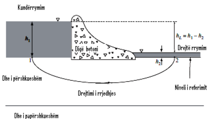
Figura 4.1. Filtrimi nëpër mjedisin poroz
