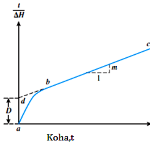
Figura 4.6 Metoda e hiperbolës për përcaktimin e c_v
