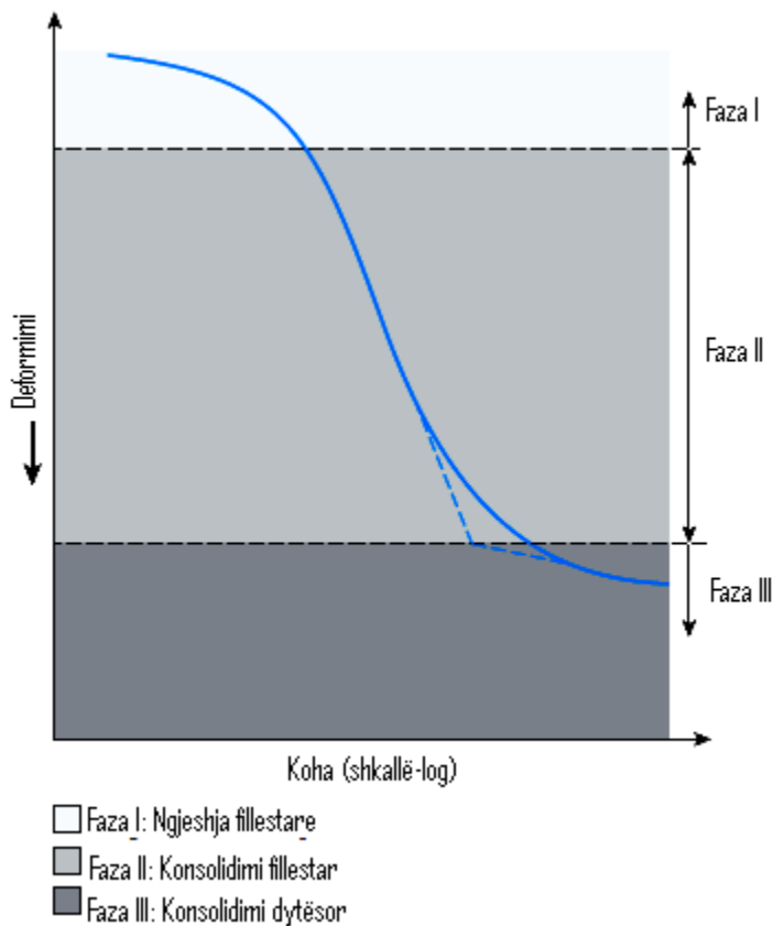
Figura 3.8 Diagrami deformim-kohë gjatë konsolidimit për rritje të caktuar të ngarkesës
