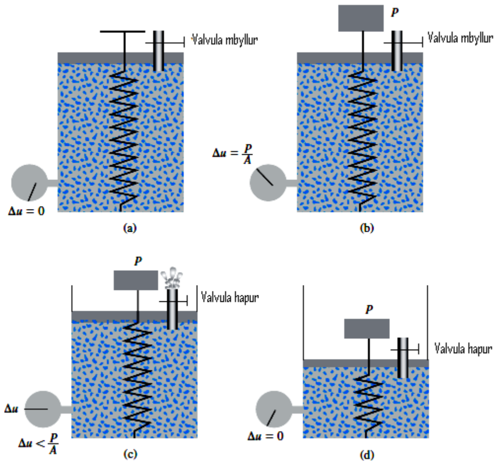
Figura 3.6 Modeli Sustë-Cilindër
