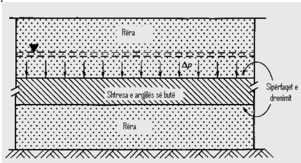
Figura 3.4. Shtresa argjilore e futur në sandviç ndërmjet shtresave ranore
