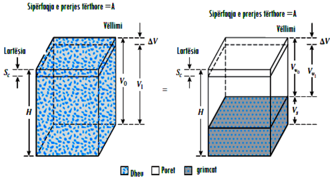
Figura 4.1 Ulja që shkaktohet nga konsolidimi njëpërmasor
