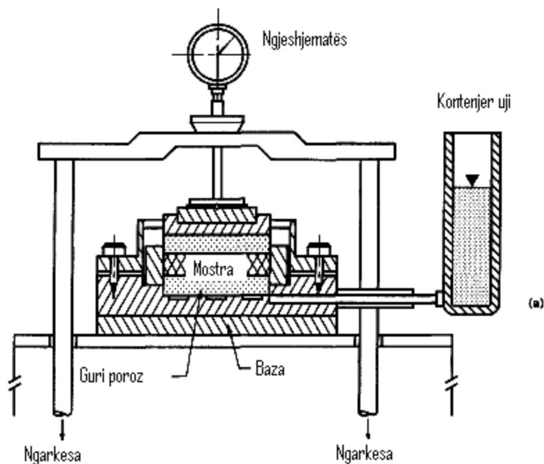
Figura 3.5 Diagrami skematik i konsolidimtatësit.(skema e aparatit eodometrik).
