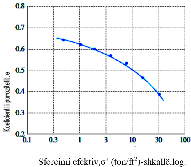
Figura 3.11 Ndryshimi i koeficientit të porozitetit në vartësi të trysnisë efektive
