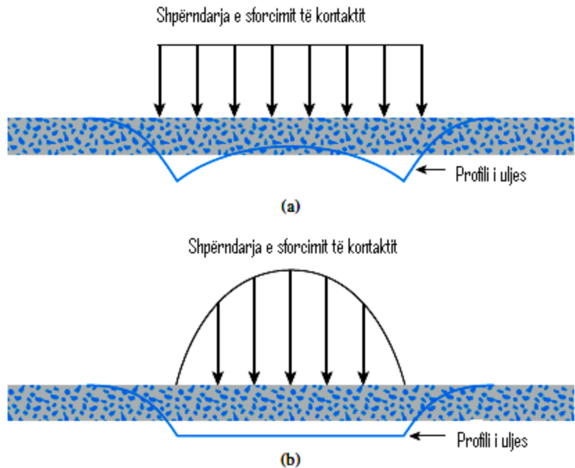
Figura 3.1. Ulja elastike e profilit dhe sforcimi i kontaktit në argjila: (a) themel elastik; (b) themel i shtangët.
