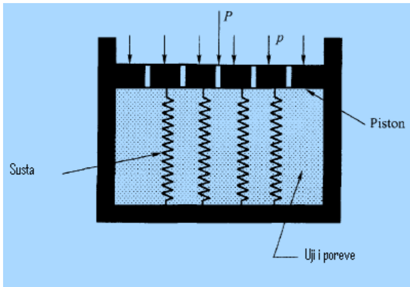
Figura 3.3. Modeli mekanik për shpjegimin e procesit të konsolidimit
