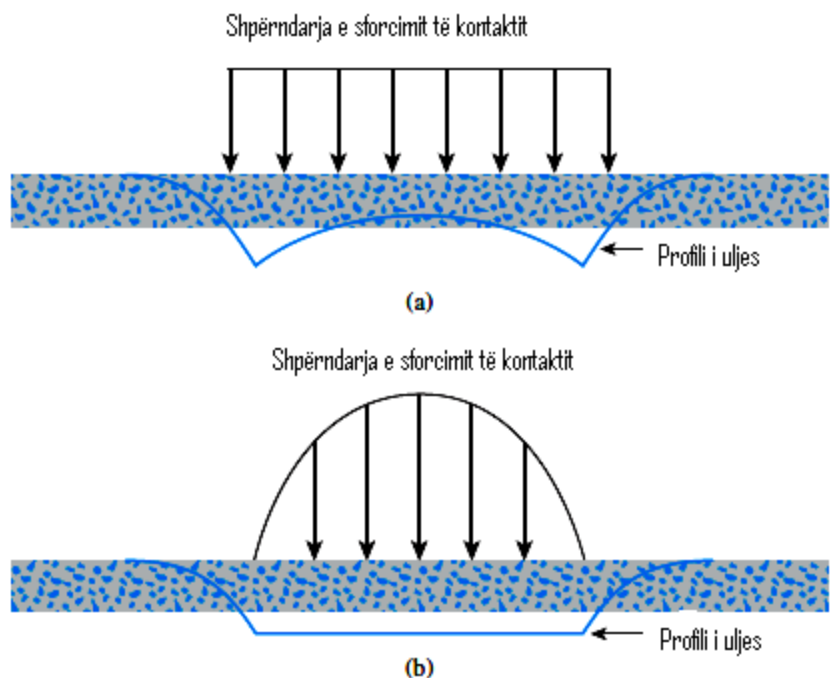
Figura 3 .2. Profili i uljes elastike dhe sforcimi i kontaktit në rrëzë; (a) themeli elastik; (b) themeli i shtangët
